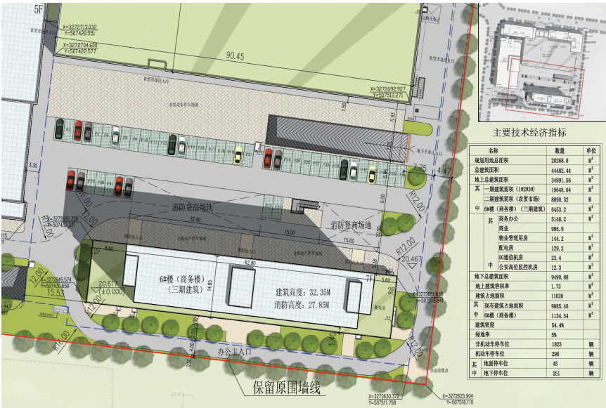
调整后总平面图
